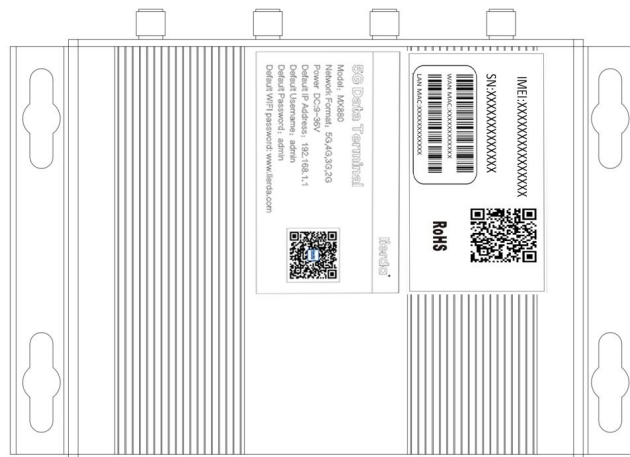
图 3-1、MX880 5G 数据终端
