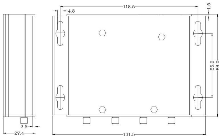
图 3-2、机械尺寸（单位：mm）
