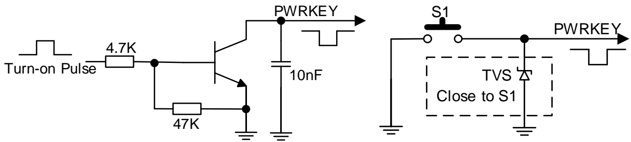
图 3.5 开关机电路
