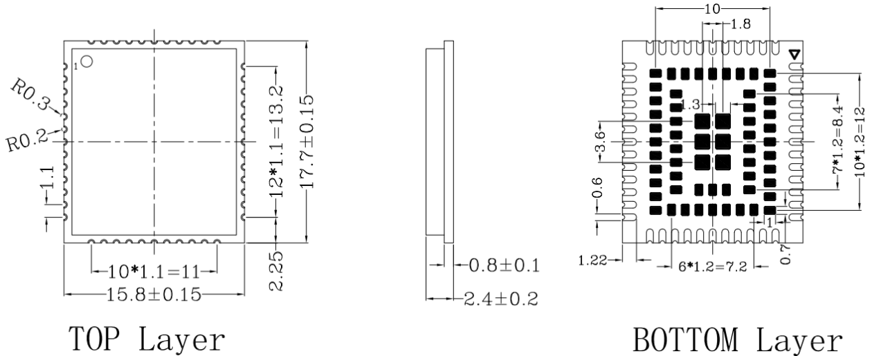
图 7.1 模组机械尺寸图(单位 mm)
