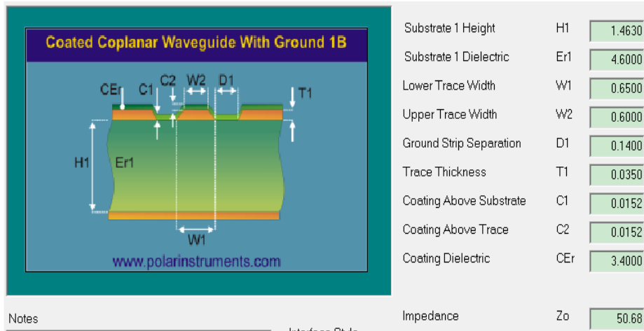
图 5.2 50 欧姆阻抗的计算方法参考
