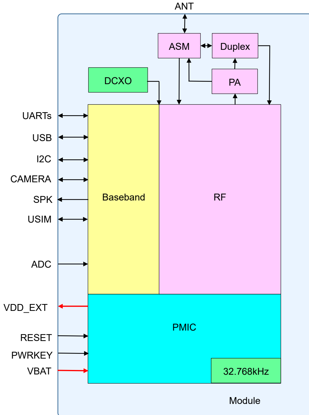
图 2.1 模组功能框图
