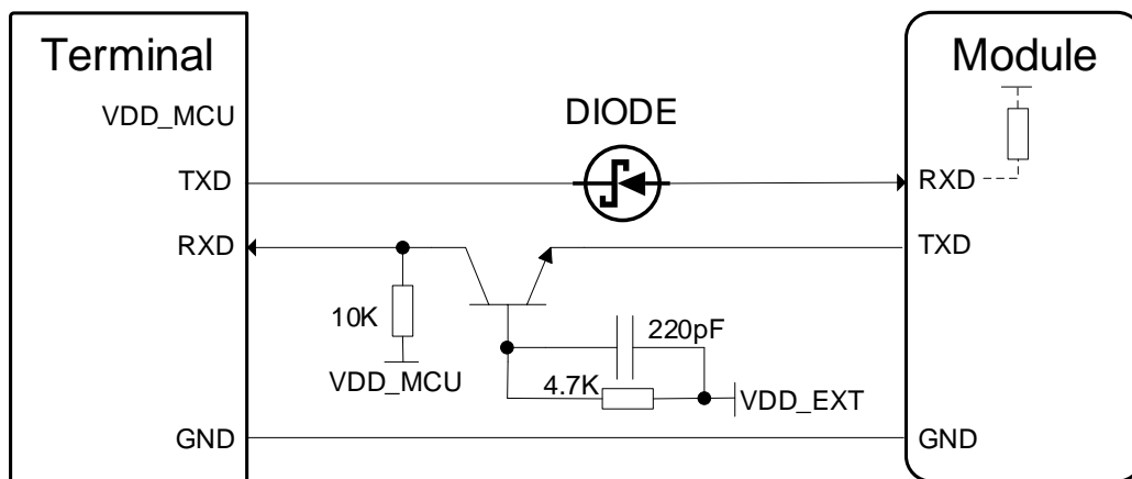
图 4.6 晶体管电平转换参考电路
