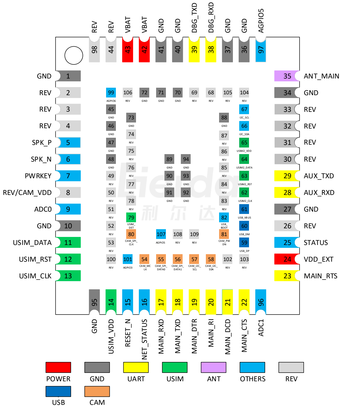
图 2.2 模组引脚分配图
