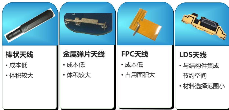
图 5.4 CAT1 常用天线类型
