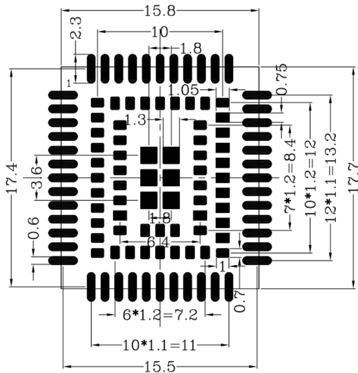
图 7.3 模组推荐焊盘(单位 mm)
