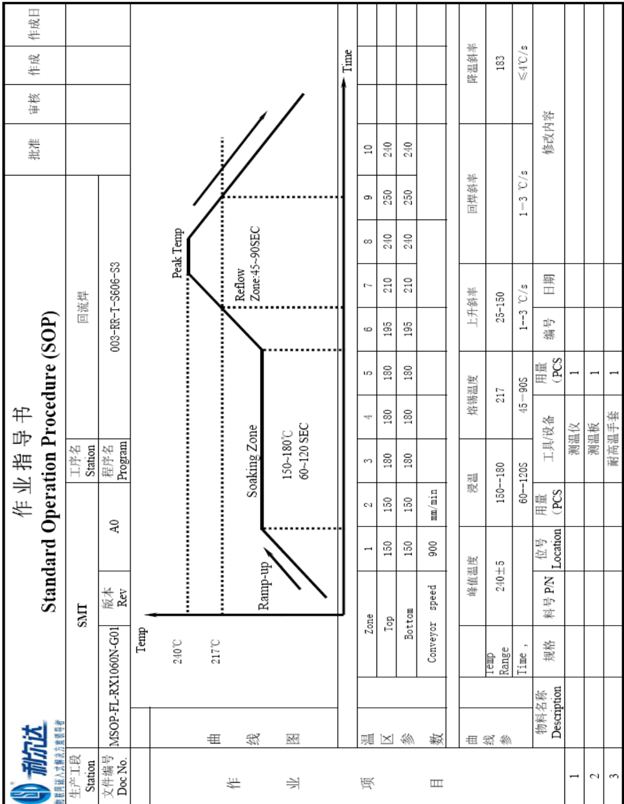
图 8.1 无铅回流焊作业指导
