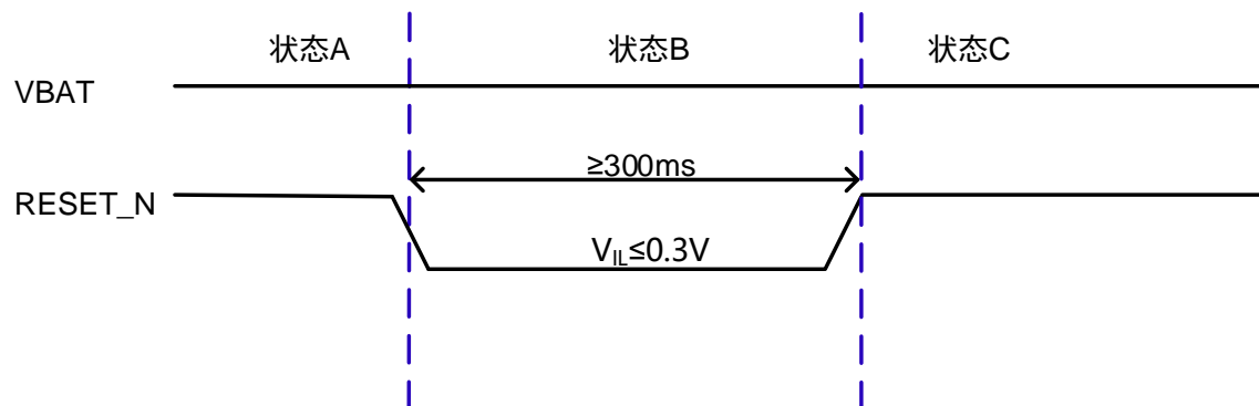
图 3.9 复位时序
